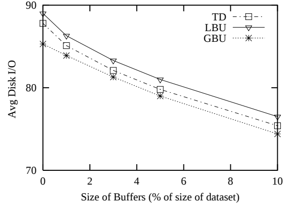
(d) Varying Buffer Size, Querying
