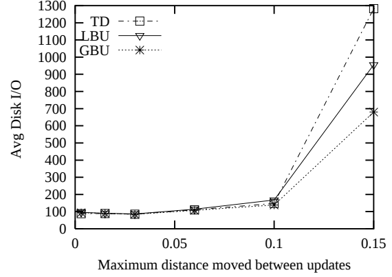
(d) Varying Maximum Distance, Querying
