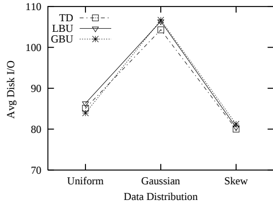
(d) Varying Data Distributions, Querying
