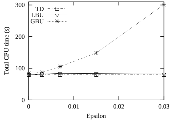
(d) Varying \epsilon : Total CPU Cost, Querying
